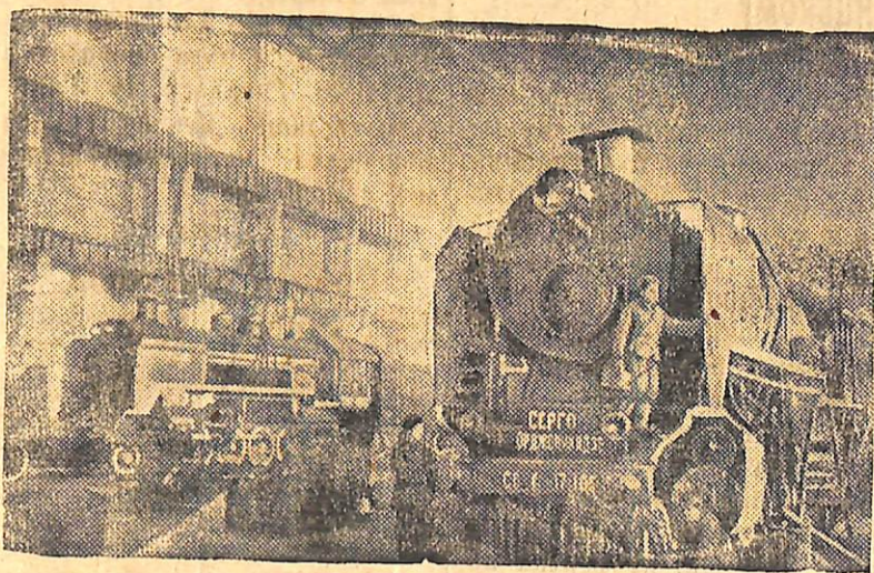
По п'ятирічному плану випуск магістральних паровозів у СРСР в 1950 р. буде доведено до 2.200. Красноярський паровозобудівельний завод успішно виконує план випуску цих паровозів. На знімку: зборка магістрального паровоза „Серго Орджонікідзе“ в цеху Красноярського заводу. Фото С. Малобицького
